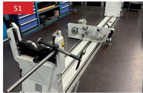
Auswuchtbank Fabrikat: CEMB HOFFMANN, Bj. 2021 Ø 500 mm x 6100 mm
