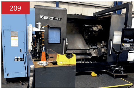
CNC-Drehzentrum Fabrikat: DOOSAN, Typ: PUMA 700M II, Bj. 2022 Ø 900 / Ø 750 x 1600 mm
